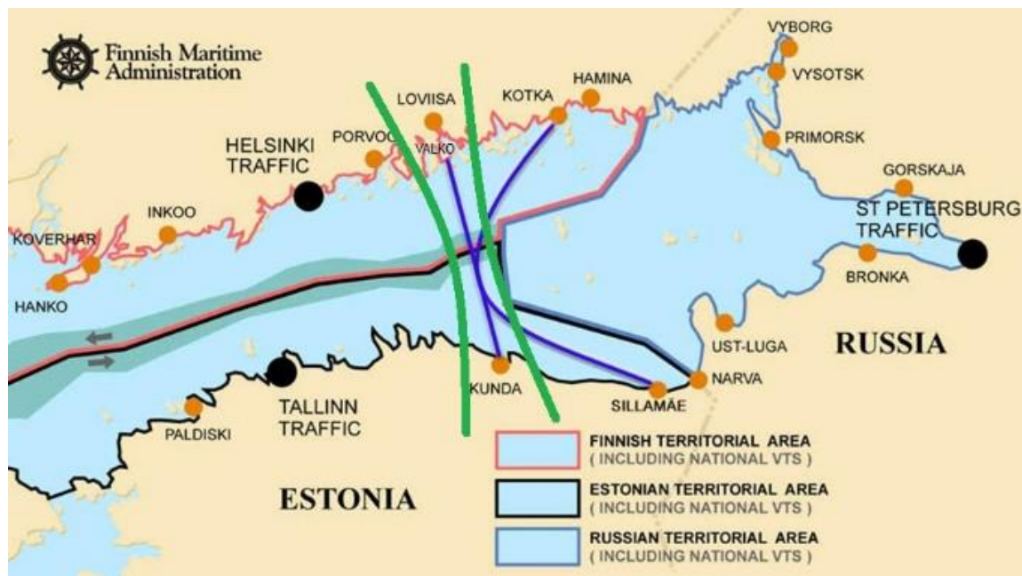
Joonis 29. Kunda-Loviisa transpordikoridori asendiplaan.
